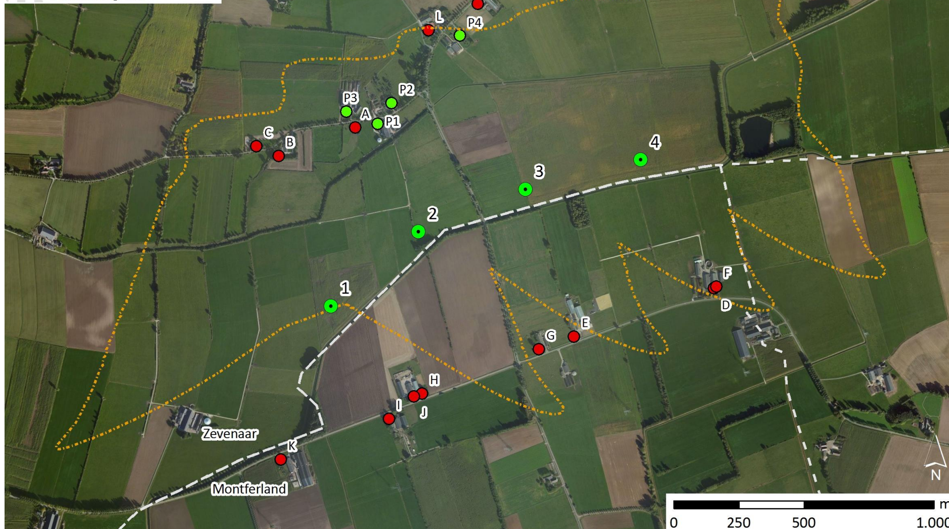
Figuur 4 – Slagschaduwcontour, rotordiameter 122m, ashoogte 124m.
